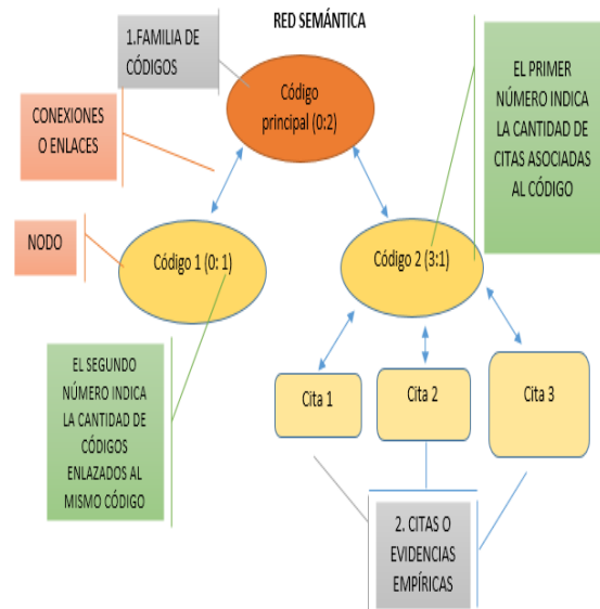
Figura 3. Red semántica
