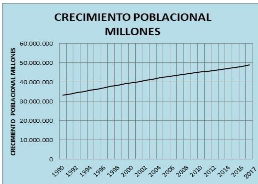
Gráfico.1 Crecimiento Poblacional
